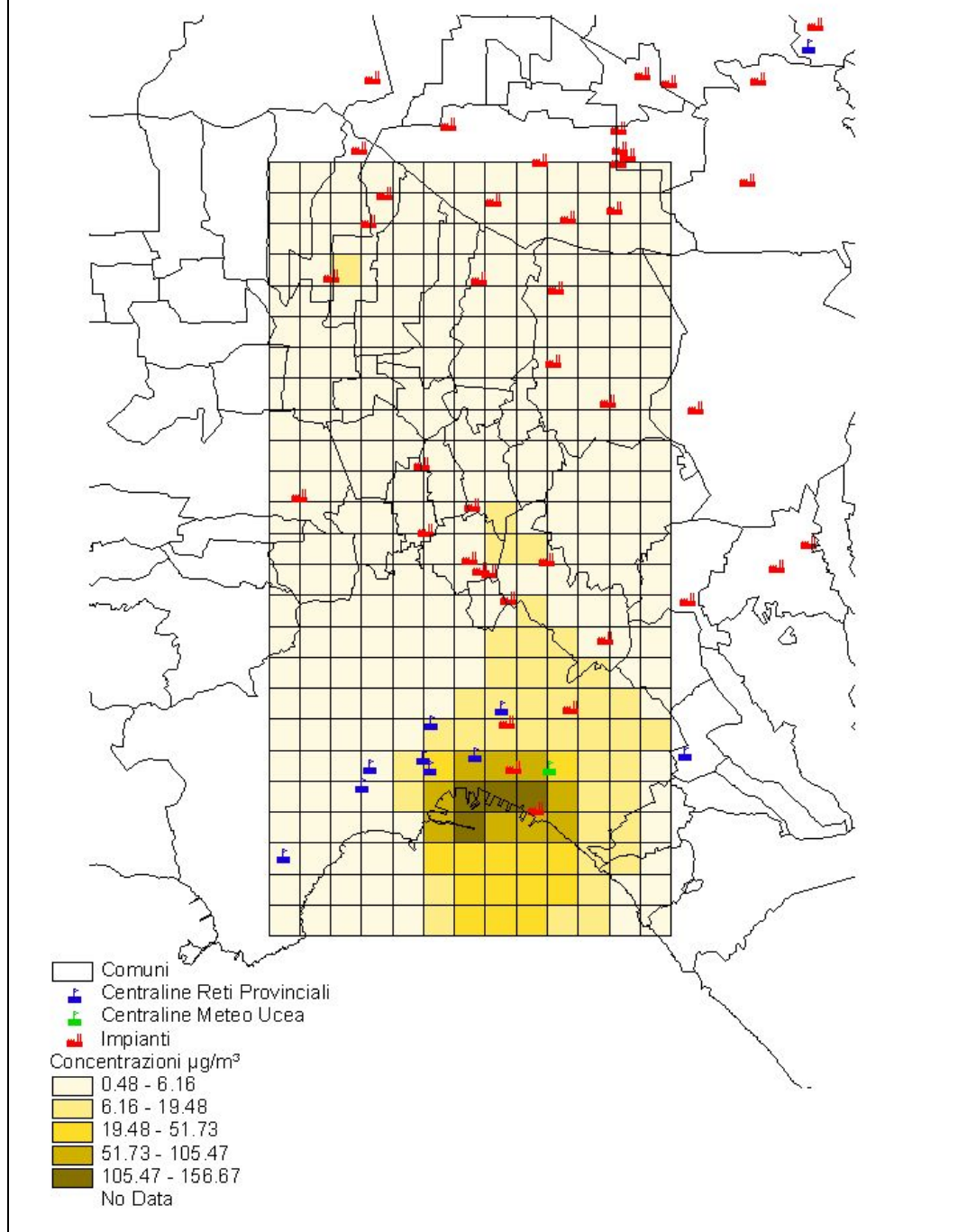
Figura 57 - Area urbana/ industriale di Napoli Caserta: concentrazioni al suolo di ossidi di zolfo calcolate mediante il modello ISC al 2010 nell'ipotesi scenario di piano (con la realizzazione di tutte le centrali termoelettriche).
