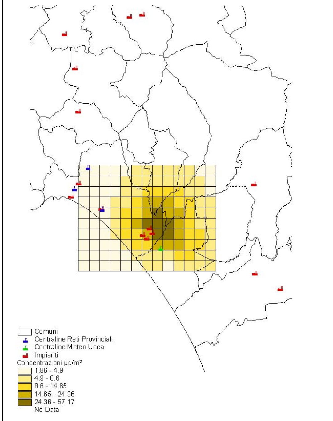
Figura 60 - Area urbana/ industriale di Salerno: concentrazioni al suolo di ossidi di zolfo calcolate mediante il modello ISC al 2010 nell'ipotesi scenario di piano (con la realizzazione di tutte le centrali termoelettriche).
