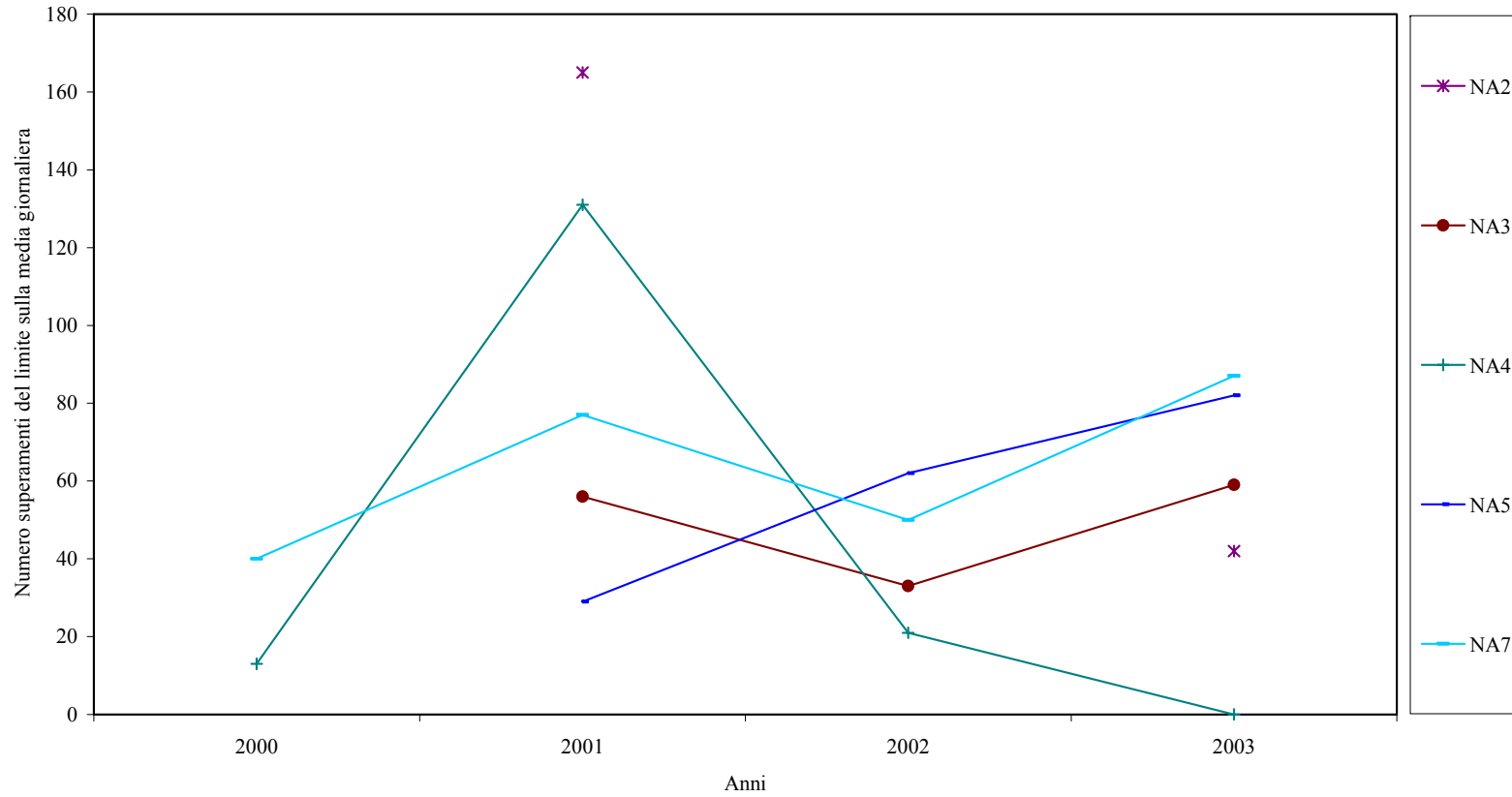
Figura 18 – Numero di superamenti della media giornaliera di particelle sospese con diametro inferiore a 10 \mu\text{m} ( \mu\text{g}/\text{m}^3 ) rilevate dalle reti di monitoraggio
