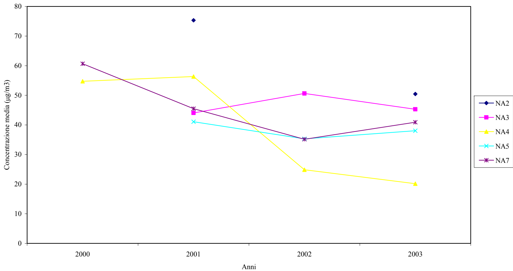
Figura 17 – Concentrazioni medie annuali di particelle sospese con diametro inferiore a 10 µm (µg/m³) rilevate dalle reti di monitoraggio
