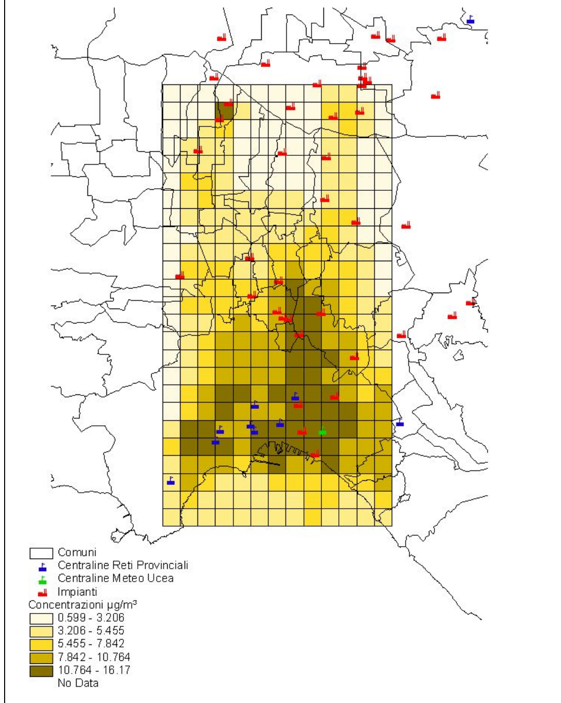
Figura 22 - Area urbana/industriale di Napoli Caserta: concentrazioni al suolo di particelle sospese con diametro inferiore a 10 \mu\text{m} calcolate mediante il modello ISC al 2002.
