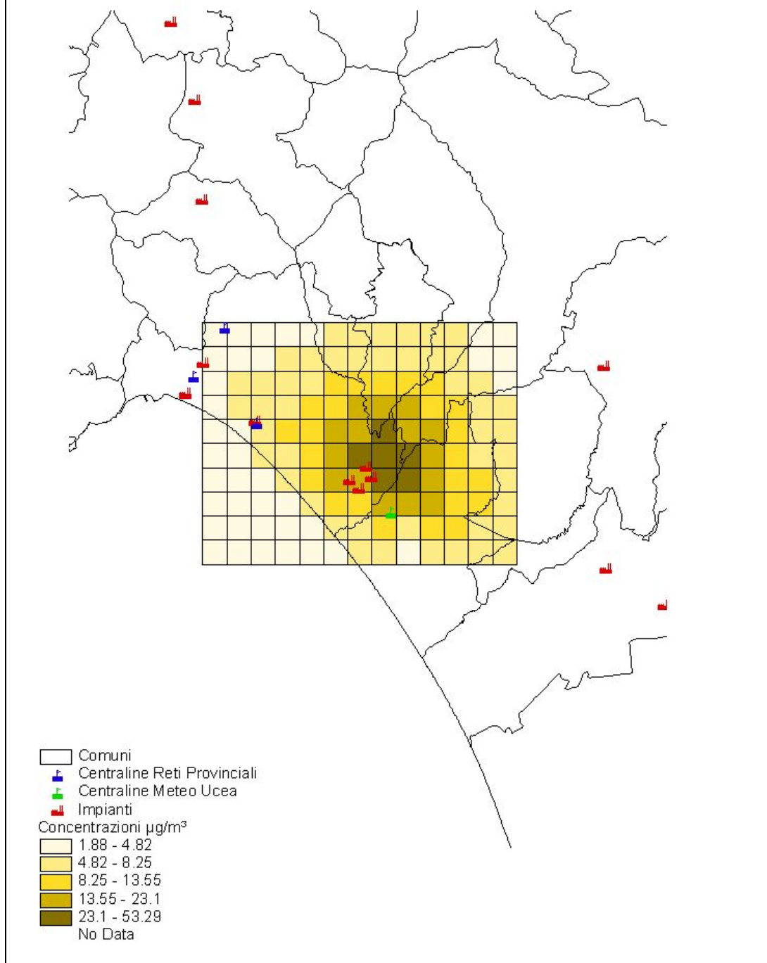
Figura 24 - Area urbana/industriale di Salerno: concentrazioni al suolo di ossidi di zolfo calcolate mediante il modello ISC al 2002.
