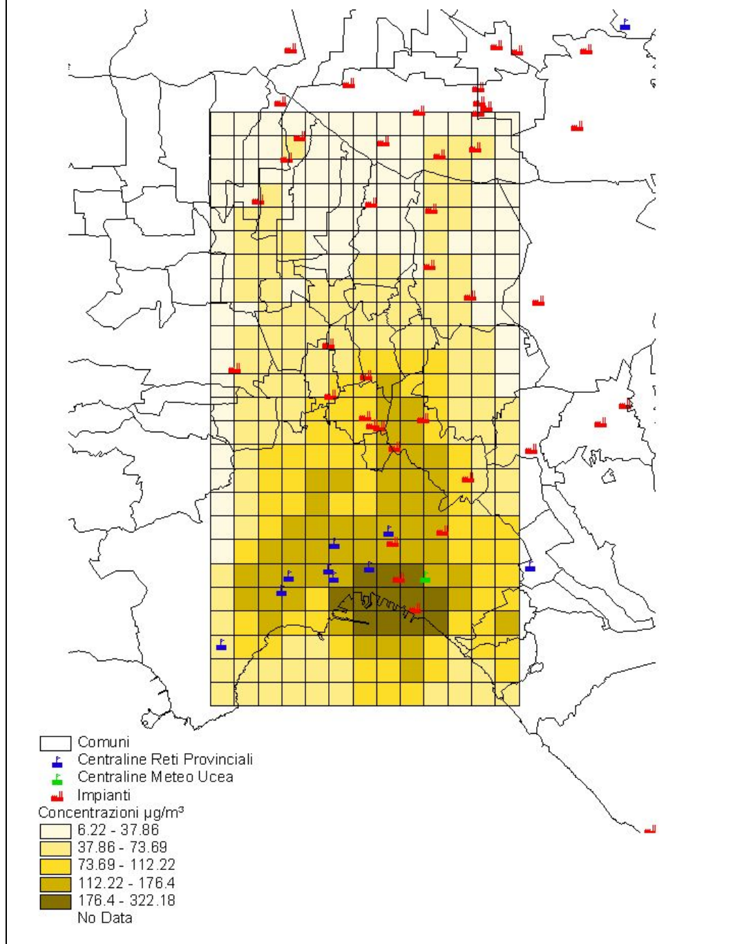
Figura 20 - Area urbana/industriale di Napoli Caserta: concentrazioni al suolo di ossidi di azoto calcolate mediante il modello ISC al 2002.
