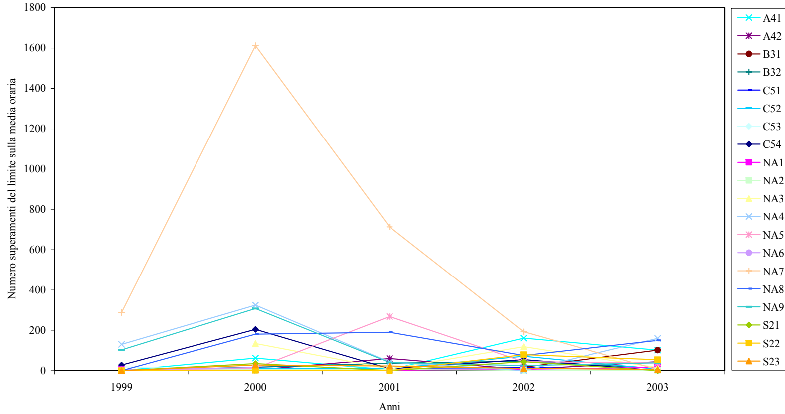
Figura 16 – Numero superamento delle medie orarie degli ossidi di azoto ( \mu\text{g}/\text{m}^3 ) rilevate dalle reti di monitoraggio
