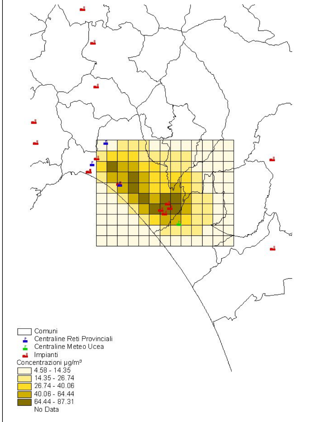
Figura 23 - Area urbana/industriale di Salerno: concentrazioni al suolo di ossidi di azoto calcolate mediante il modello ISC al 2002.
