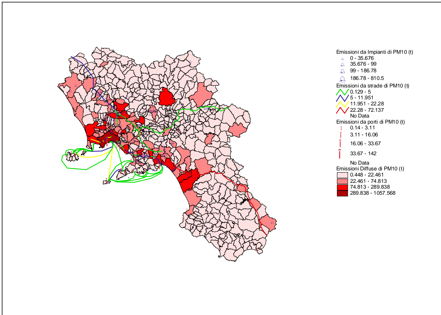
Figura 10 - Emissioni totali di particelle sospese con diametro inferiore a 10 µm – Anno 2002
