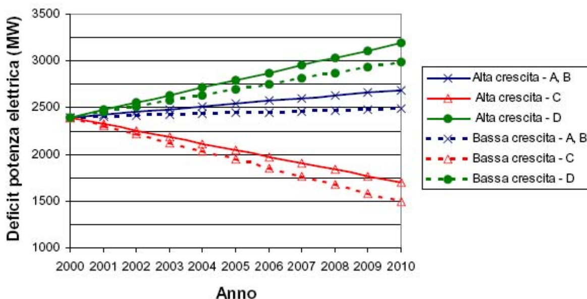
Figura 28 - Andamento del deficit di potenza elettrica in Campania. Scenari di tendenza 2000 – 2010
