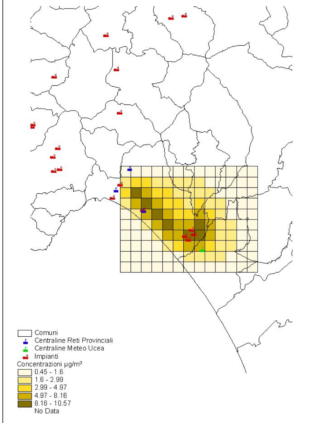
Figura 25 - Area urbana/industriale di Salerno: concentrazioni al suolo di particelle sospese con diametro inferiore a 10\ \mu\text{m} calcolate mediante il modello ISC al 2002.
