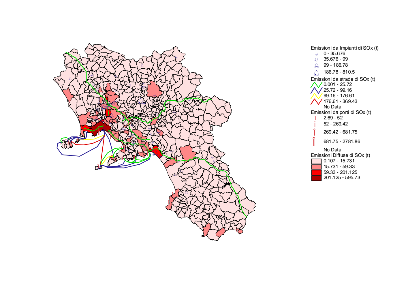
Figura 6 - Emissioni totali di ossidi di zolfo – Anno 2002
