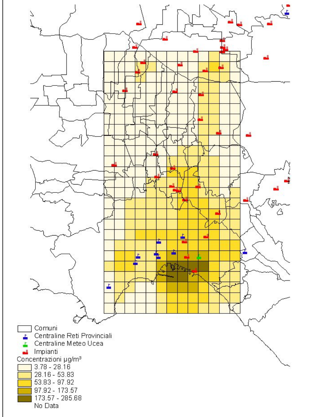
Figura 43 - Area urbana/ industriale di Napoli Caserta: concentrazioni al suolo di ossidi di azoto calcolate mediante il modello ISC al 2010 nell'ipotesi in assenza di interventi.
