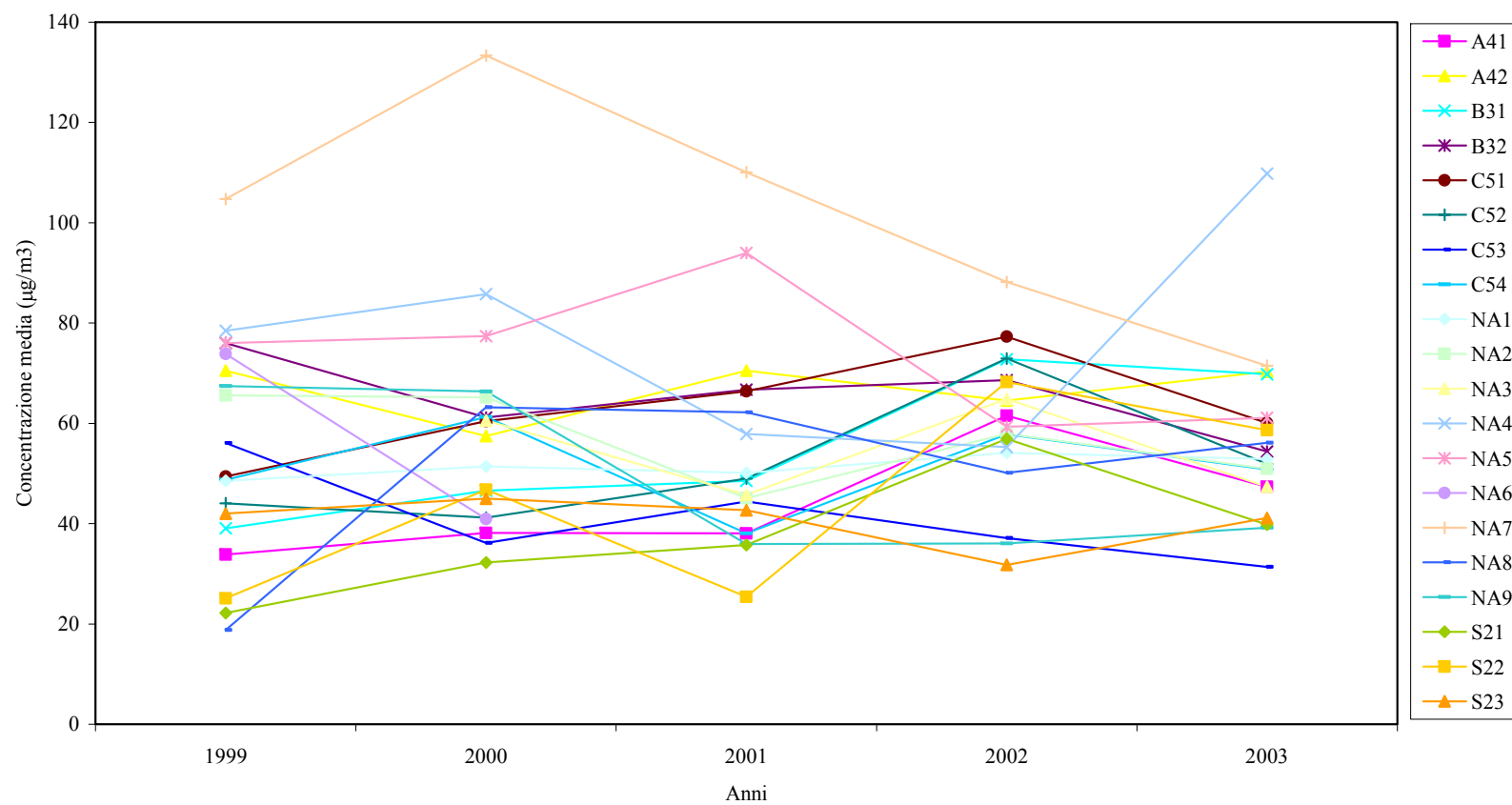
Figura 15 – Concentrazioni medie annuali degli ossidi di azoto ( \mu\text{g}/\text{m}^3 ) rilevate dalle reti di monitoraggio
