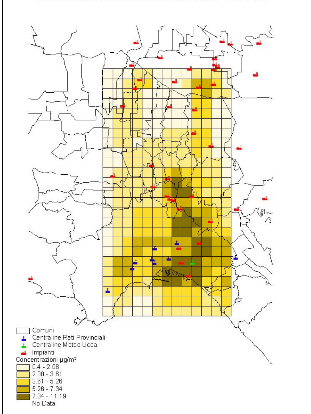
Figura 58 - Area urbana/ industriale di Napoli Caserta: concentrazioni al suolo di particelle sospese con diametro inferiore a 10 \mu\text{m} calcolate mediante il modello ISC al 2010 nell'ipotesi scenario di piano (con la realizzazione di tutte le centrali termoelettriche).
