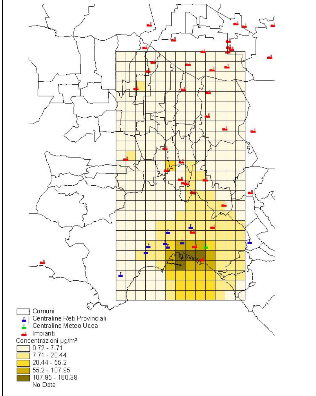
Figura 21 - Area urbana/industriale di Napoli Caserta: concentrazioni al suolo di ossidi di zolfo calcolate mediante il modello ISC al 2002.
