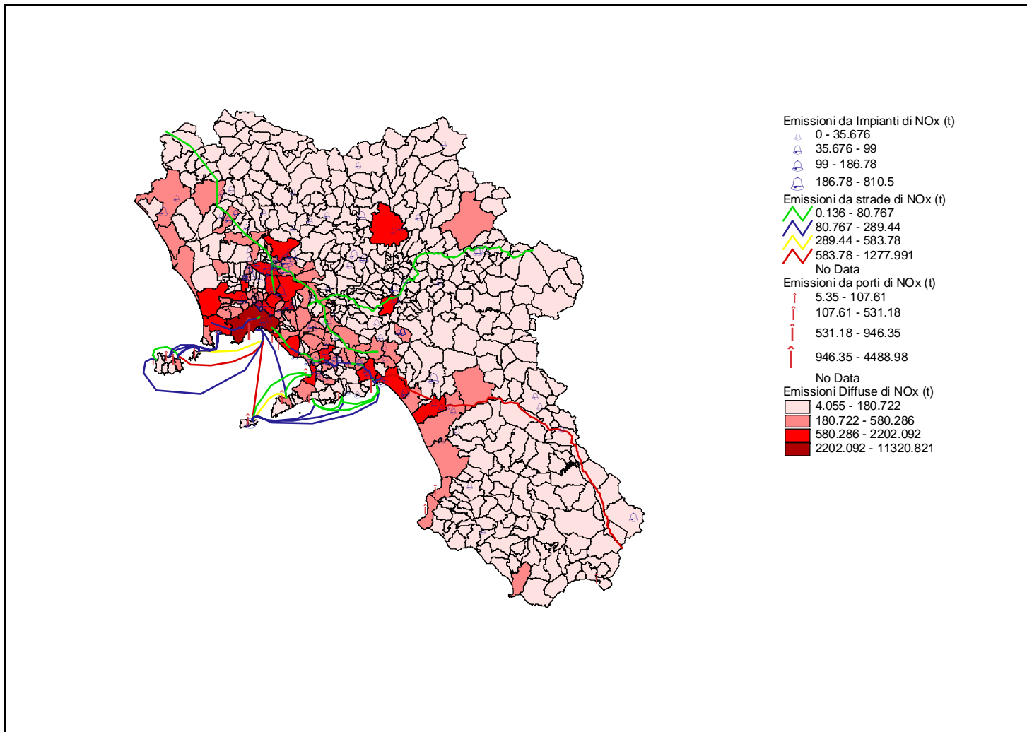
Figura 7 - Emissioni totali di ossidi di azoto – Anno 2002
