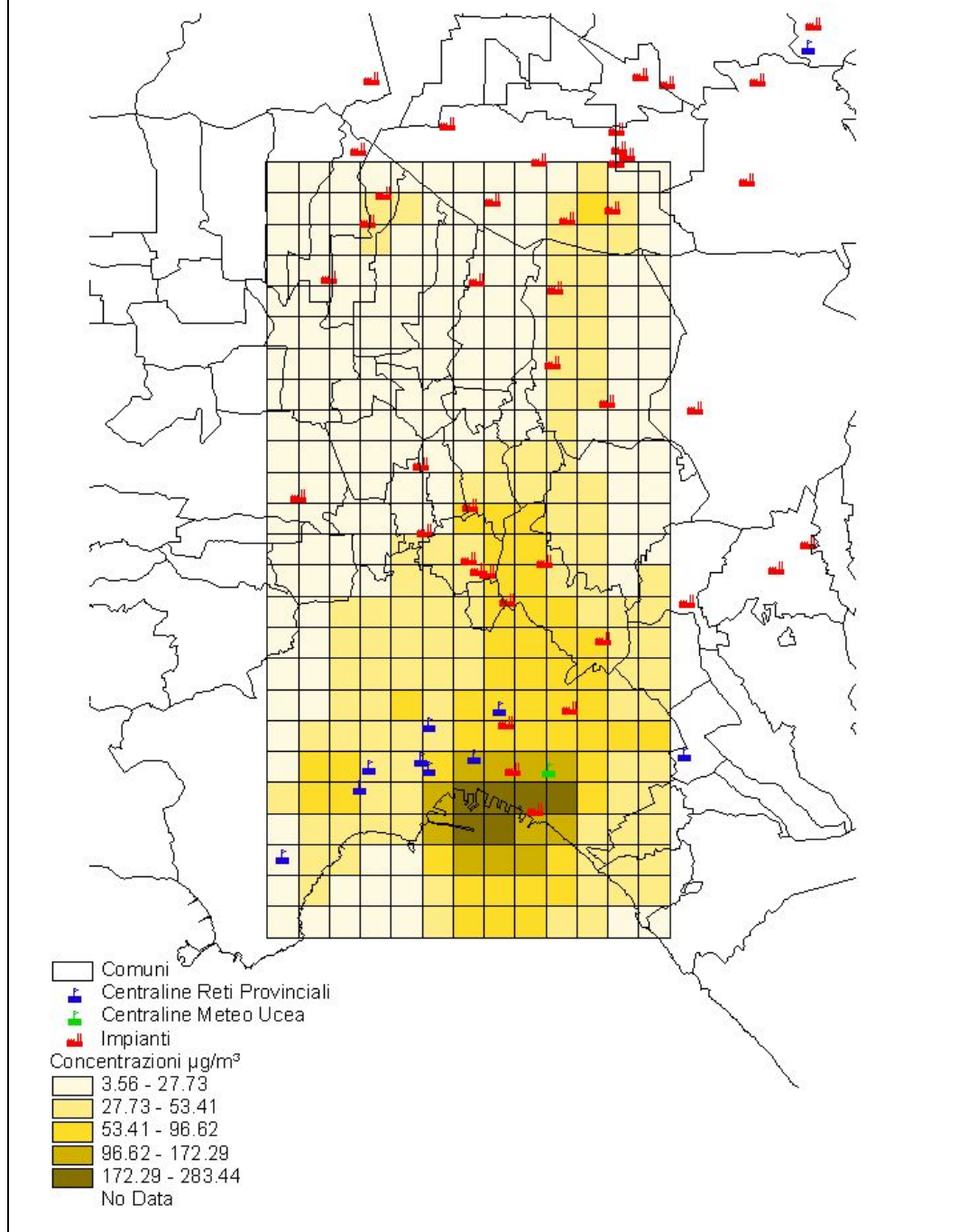
Figura 56 - Area urbana/ industriale di Napoli Caserta: concentrazioni al suolo di ossidi di azoto calcolate mediante il modello ISC al 2010 nell'ipotesi scenario di piano (con la realizzazione di tutte le centrali termoelettriche).
