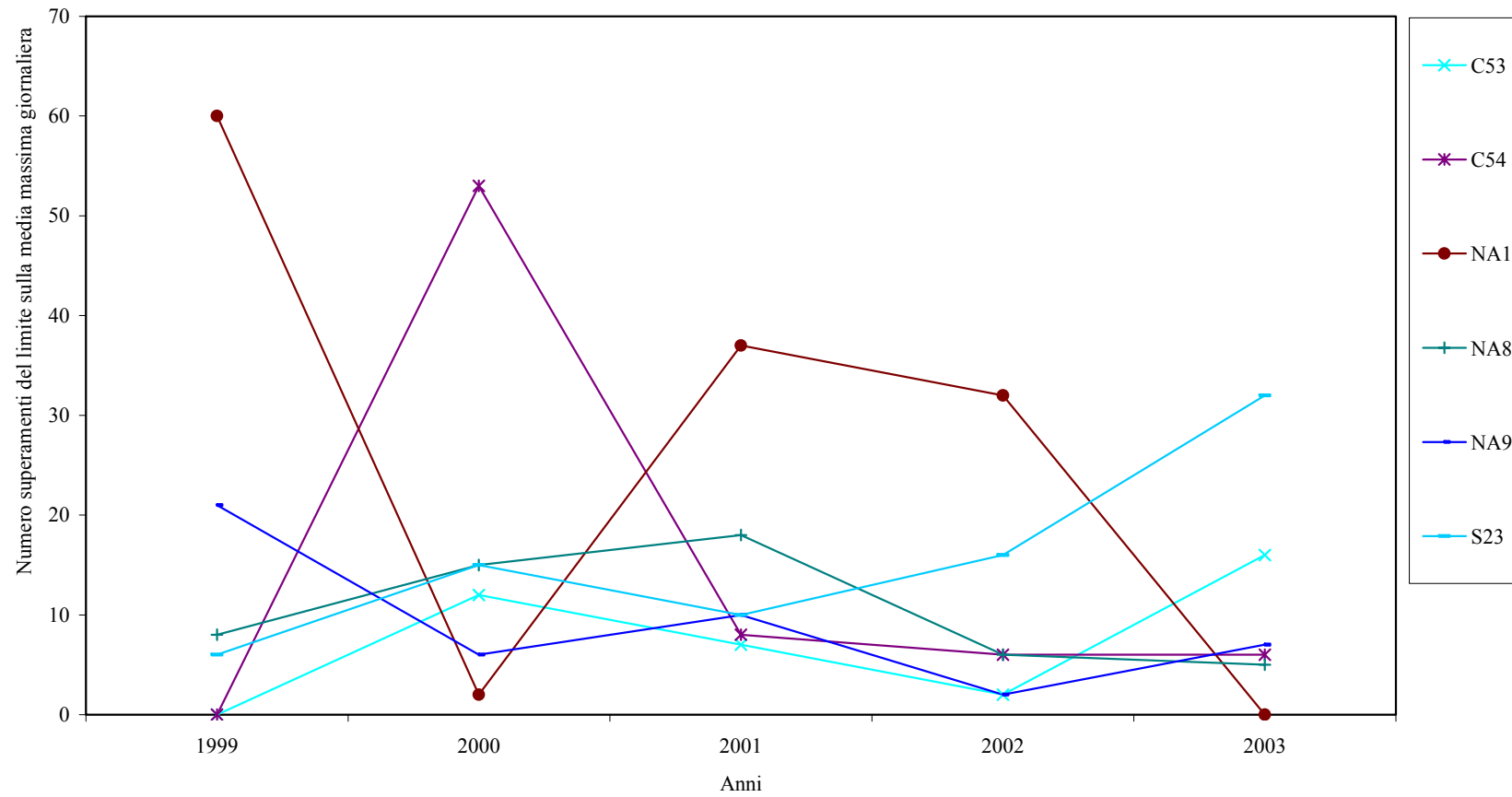
Figura 19 – Ozono: numero di superamenti della media su 8 ore ( 120 \mu\text{g}/\text{m}^3 ) rilevate dalle reti di monitoraggio
