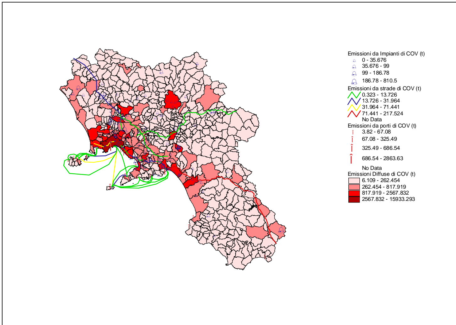
Figura 9 - Emissioni totali di composti organici volatili – Anno 2002
