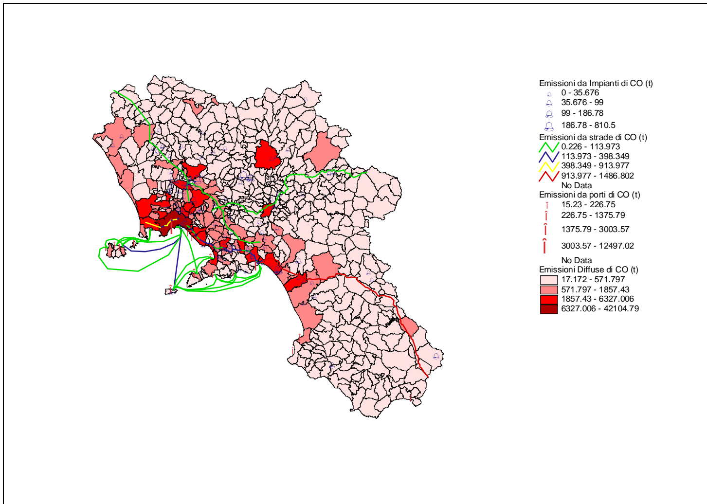
Figura 8 - Emissioni totali di monossido di carbonio – Anno 2002
