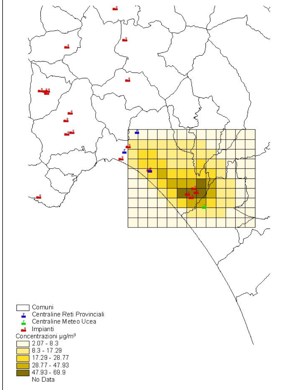
Figura 59 - Area urbana/ industriale di Salerno: concentrazioni al suolo di ossidi di azoto calcolate mediante il modello ISC al 2010 nell'ipotesi scenario di piano (con la realizzazione di tutte le centrali termoelettriche).
